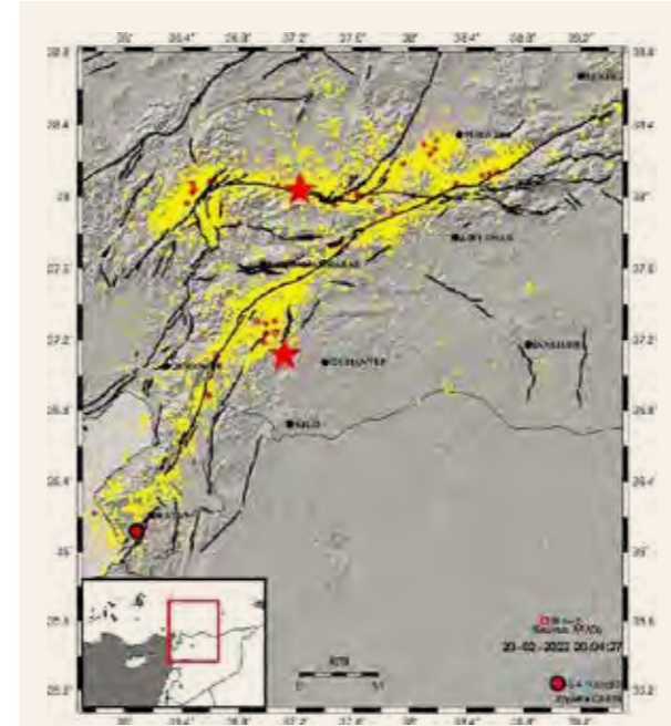
Görüntü 2. Onbiril Depremi, sarsıntı odakları (yıldızlar) ile etkileme alanları, kırılan yerlerdeki çatlaklar (faylar).
