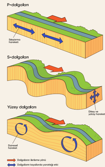
Görüntü 3. Deprem gerginliğinin bir kırıkla boşalması ile işleyişi: kırık çizgisi, kırık düzlemi, deprem odağı (hypocenter), deprem dış odağı (epicenter), odaktan üreyen sarsım dalgaları (solda). Sarsıntı dalgalarının ardı ardına üç türlü, ilerleyerek size doğru gelişi: derinden gelen P-sıkıştırma-açma-kalıtma dalgası, S-sağa sola burkma dalgası, yüzey dalgaları, L-çalkalama (love), R-ters çevirme, itip-çekme, döndürme dalgası (Raileigh).
